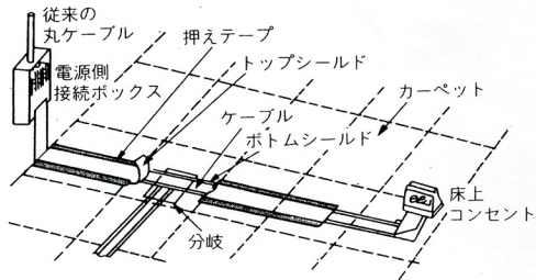
第2図 アンダーカーペット配線方式—某社製
