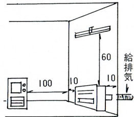
密閉式石油ストーブ
