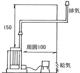
半密閉式石油ストーブ
