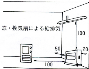
開放式石油ストーブ
