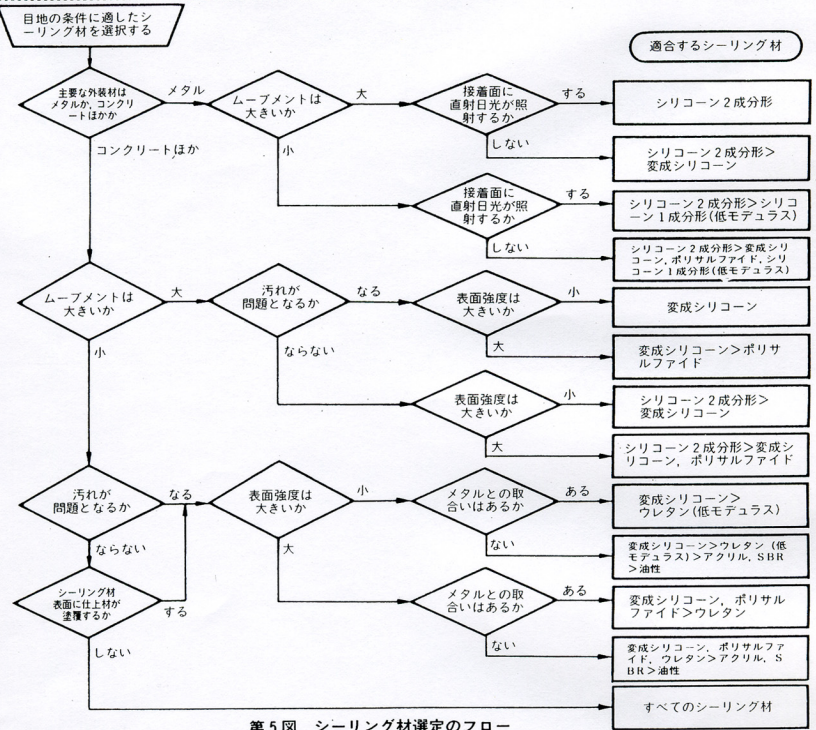
第5図 シーリング材選定のフロー
